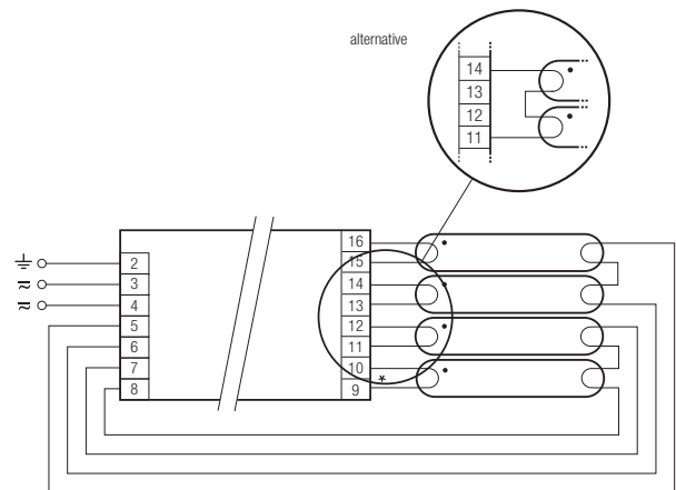
PC 2/14-21-28-35 T5 PRO Ip
