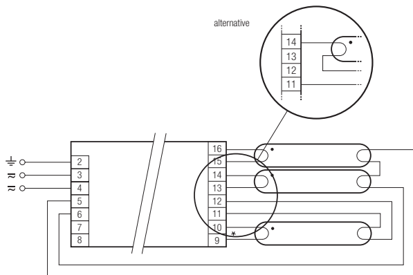
PC 1/14-21-28-35 T5 PRO Ip
