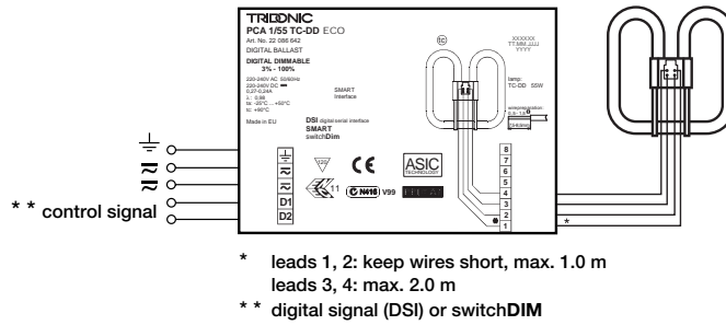
PCA TC-DD ECO 55 W
